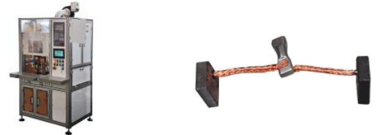
Soldador MFDC de 110KVA para arrancador de coche DB-110-15010
